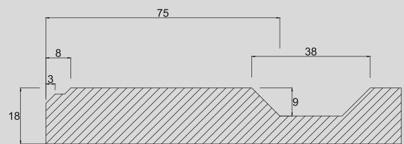
Przekrój
