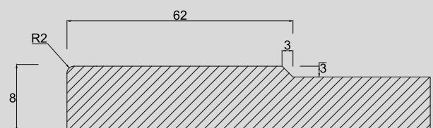
Przekrój
