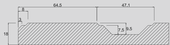
Przekrój
